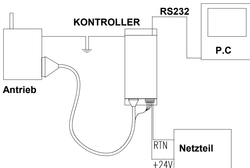
Bild 4: Erdungsanordnung
